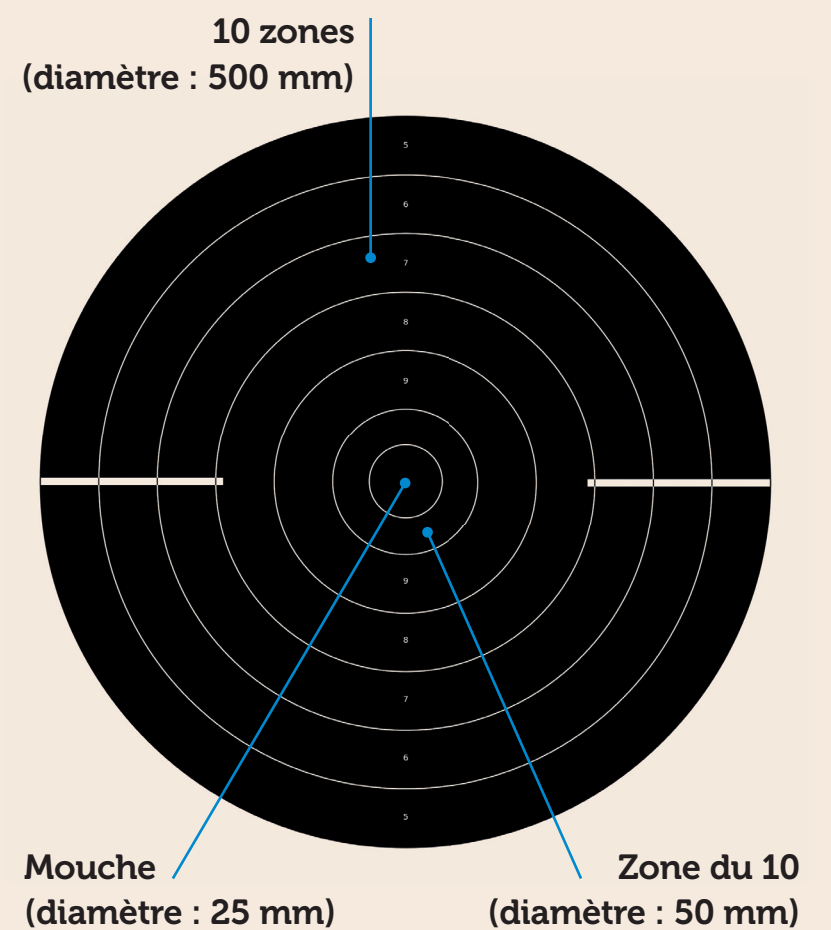
Cible pistolet 25 m (vitesse)
